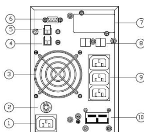
а. 8S Power U1001TS1 задняя панель
