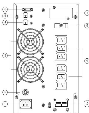
б. 8S Power U1002TS1 & U1003TS1 задняя панель
