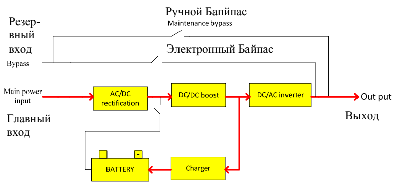
Рисунок 1.3 Схема рабочего процесса в сетевом рабочем режиме ИБП.
