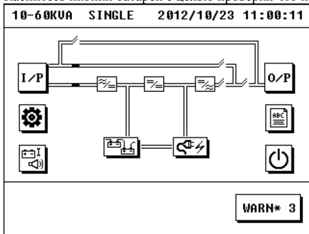
Рисунок 3.11 Главный интерфейс
