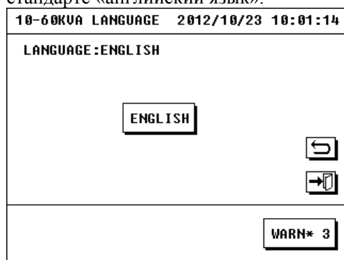
Рисунок 3.38 Экран языка
