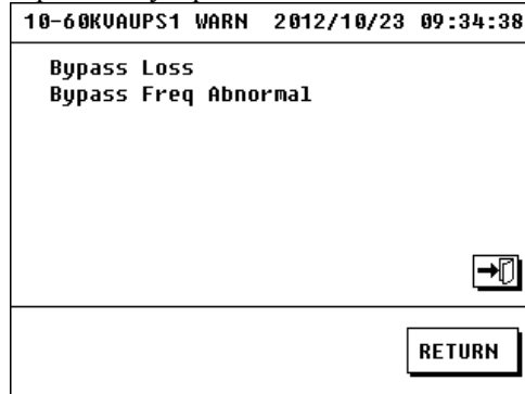
Рисунок 3.26 Интерфейс предупреждений
