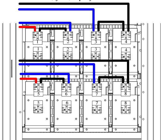
Рисунок 2.15 Схема подключения батарейного блока
