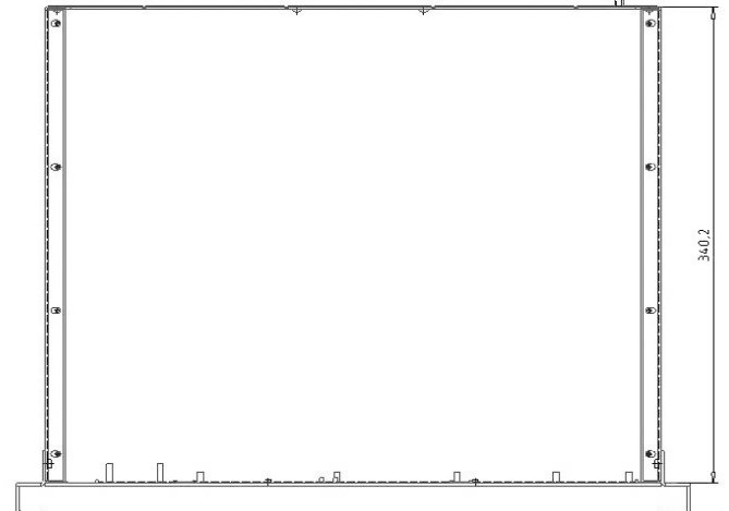
Инвертор PS220/700C-P-2
