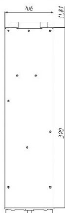
Инвертор PS48-60/2000K, PS48-60/2000K(I)
