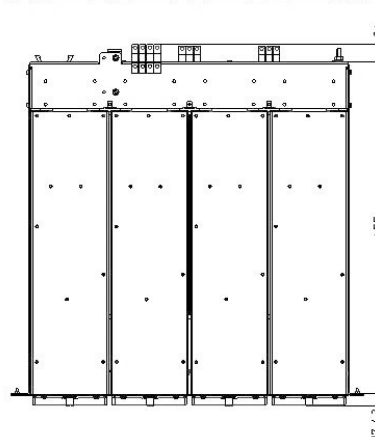
Модульный каркас PS2000K с 4-мя инверторами PS48-60/2000K
