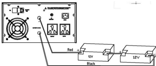
ИБП 1600W - 24V, подключение батарей (Красный кабель подключается к «+» батареи, черный кабель подключается к «-» батареи)
