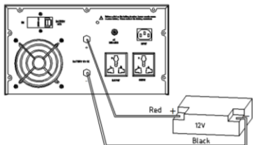
ИБП 300W / 600W / 1000W - 12V, подключение батарей (Красный кабель подключается к «+» батареи, черный кабель подключается к «-» батареи)
