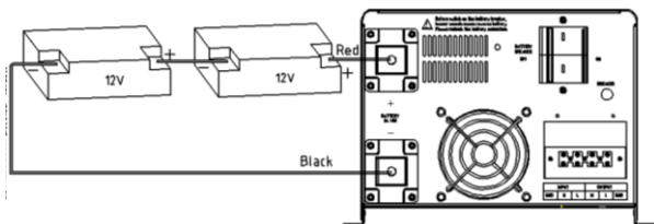
ИБП 2500W / 3500W - 24V подключение батарей (Красный кабель подключается к «+» батареи, черный кабель подключается к «-» батареи. Для модели 2500W батарейный кабель должен иметь сечение >35mm 2 , 3500W - должен иметь сечение >50mm 2 )
