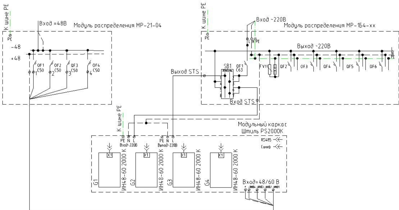
Инверторы Штиль PS48-60/2000K в модульном каркасе PS2000K с модулями распределения
