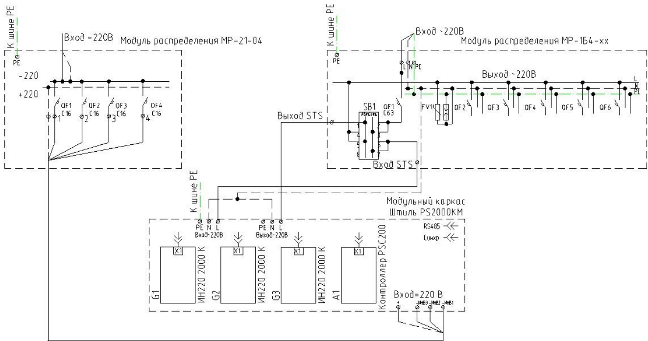
Инверторы Штиль PS220/2000K с контроллером Штиль PSC-200.03.02 в модульном каркасе PS2000KM, с модулями распределения
