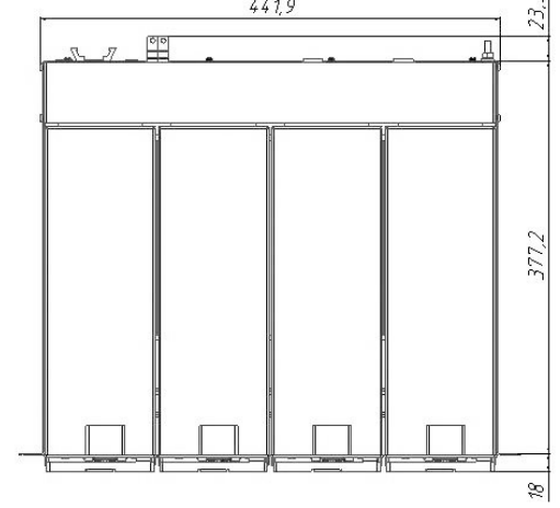
Модульный каркас PS500K с 4-мя инверторами PS48-60/500K
