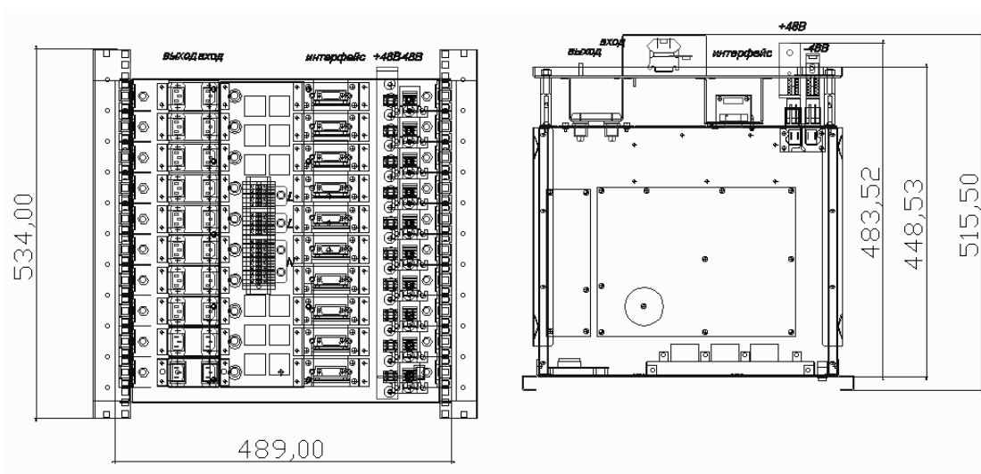
Модульный каркас Штиль PSI10/1500
