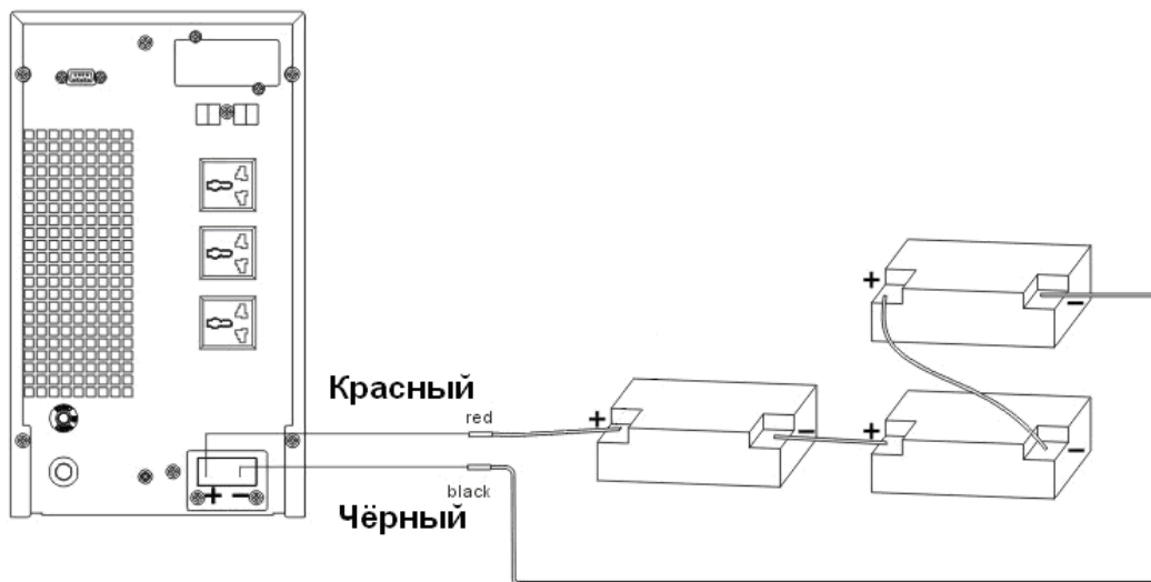
ИБП RVBMP 1кВА LT. Подключение батарей.(3АКБ послед.) Схема сборки батарей относится к ИБП с корпусом RT и TOWER.
