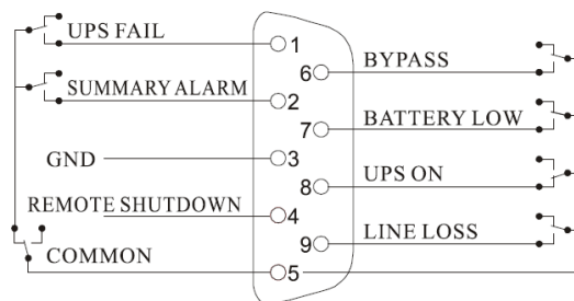
Рис. DB-9 Интерфейс AS400
