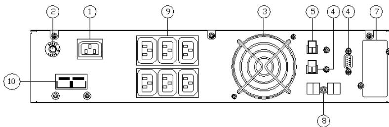
с. ИБП 1кВА-RT (24В внутр.АКБ) ; 1кВА-RT (36В LT) [ИБП 1кВА-RT (36В внутр.АКБ) опция ]
