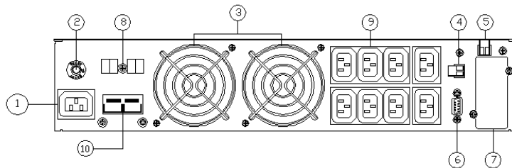
д. ИБП 2кВА-RT (48В внутр.АКБ); 3кВА-RT (72В внутр.АКБ) [ИБП 2кВА-RT (72В внутр.АКБ) опция ]
