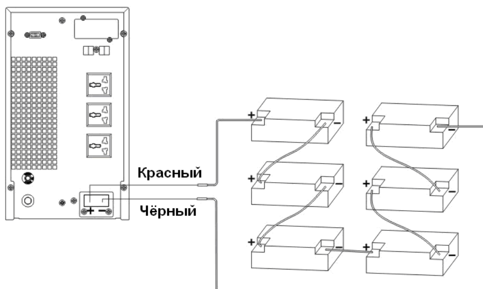
ИБП RVBMP 2кВА LT. Подключение батарей. (6АКБ послед.) Схема сборки батарей относится к ИБП с корпусом RT и TOWER.
