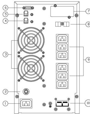
б. ИБП 2кВА, 3кВА (внутр.АКБ / LT) [ИБП 2,3кВА опция]
