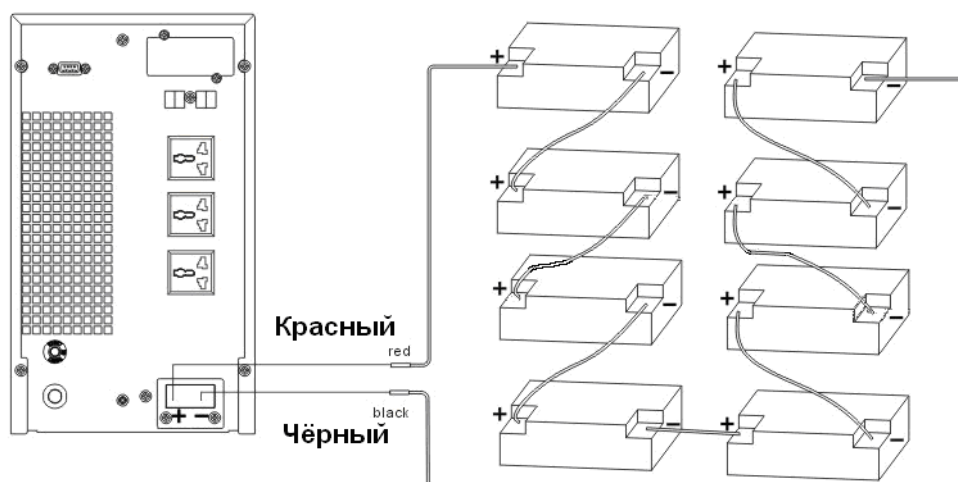
ИБП RVBMP 3кВА LT. Подключение батарей. (8АКБ послед.) Схема сборки батарей относится к ИБП с корпусом RT и TOWER.
