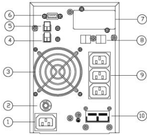
а. ИБП 1кВА (внутр.АКБ / LT) [ИБП 1кВА опция]
