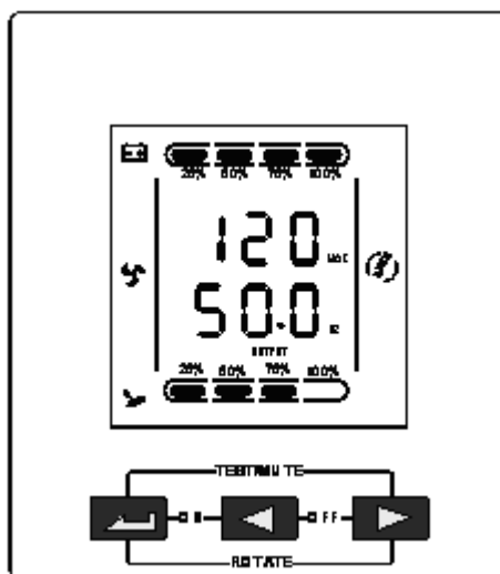
экран стоечной модели RT.
