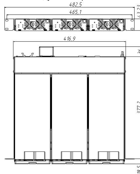
Модульный каркас PS1000K
