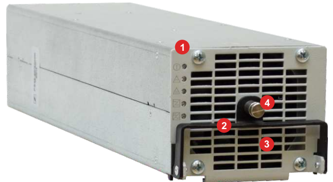
Инвертор Штиль PS48-60/2000K(I)
