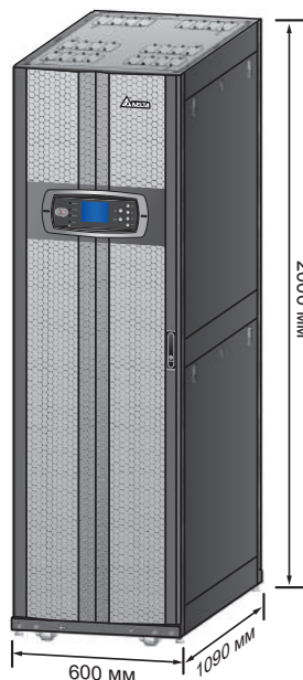
Рис. 2-2. Размеры
