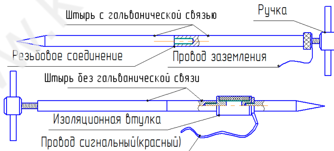
Рис.2. Штыри в сборе
