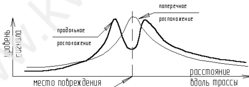
Рис.9. Изменение сигнала при обследовании изоляции
