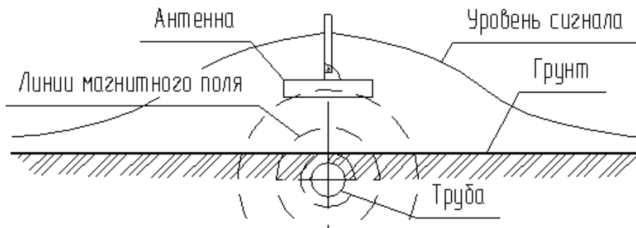
Рис.6. Определение оси трассы по максимуму
