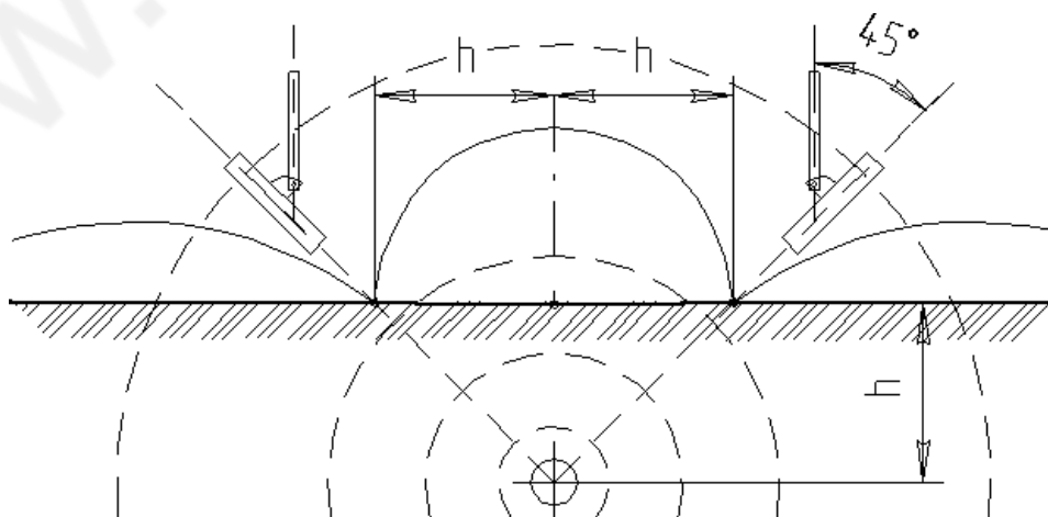
Рис.8. Определение глубины методом 45 градусов
