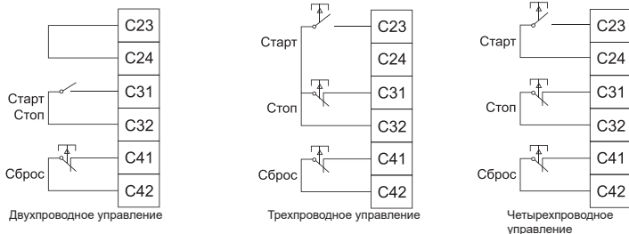
Рисунок 3 – Схемы управления
