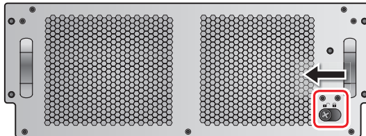
Рис. 5-28. Разблокировка защёлки
