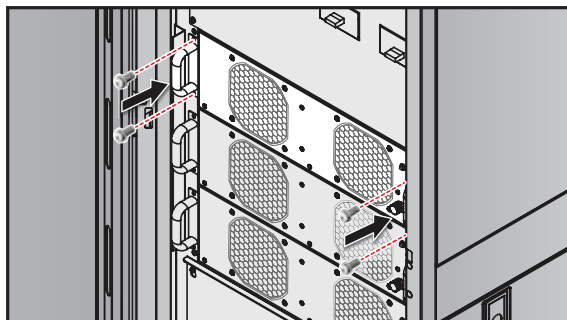
Рис. 5-21. Фиксация винтами
