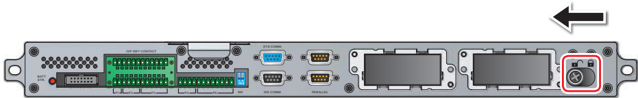
Рис. 5-31. Разблокировка защёлки
