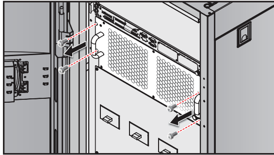
Рис. 5-29. Выкручивание винтов
