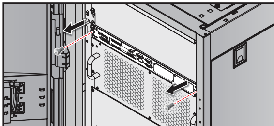
Рис. 5-32. Выкручивание винтов
