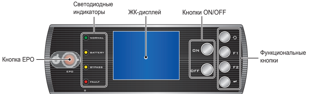
Рис. 7-2. Панель управления
