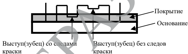
Рисунок 1 – Проведение испытания
