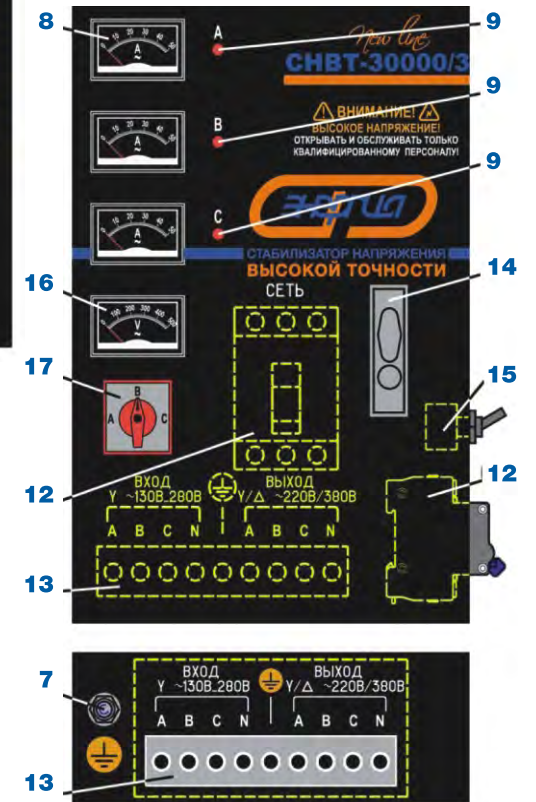
Рис. 7. Модели SNVT-9000/3...60000/3 Передняя панель – сверху. Задняя панель – внизу.
