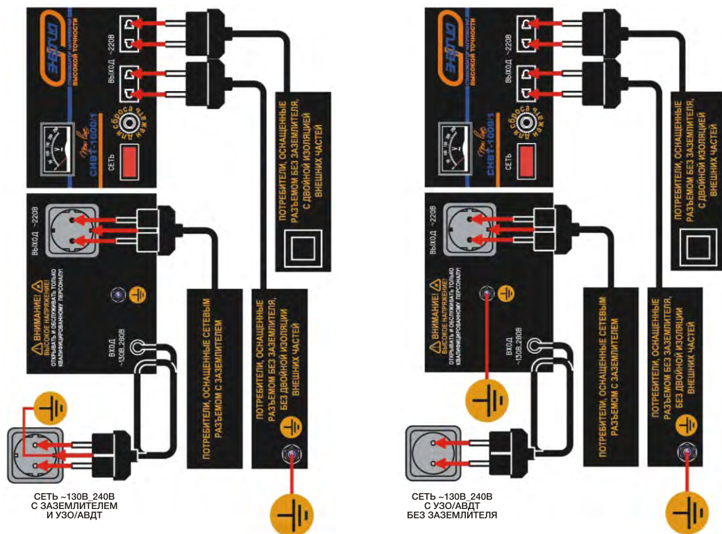
Рис. 8. Требования электробезопасности при подключении.
