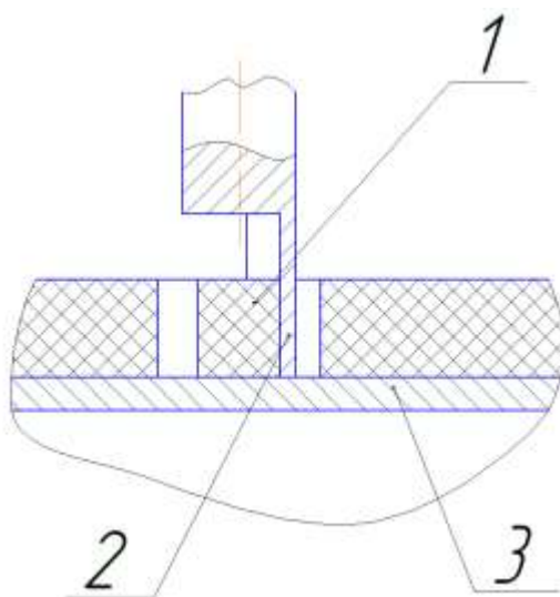
Рис. 9 Схема установки измерителя при определении адгезии битумного покрытия 1 - вырезанный образец, 2 – штук, 3 – труба
