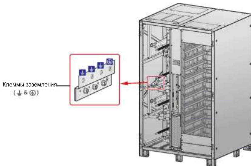
Рисунок 2-9: Клеммы заземления
