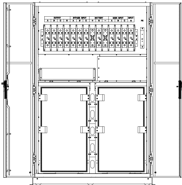
(е) модели ИБП 400 кВА и 500 кВА Рисунок 1-8внешний вид ИБП
