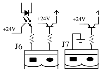
Рисунок 2-14Разъем ВСВ
