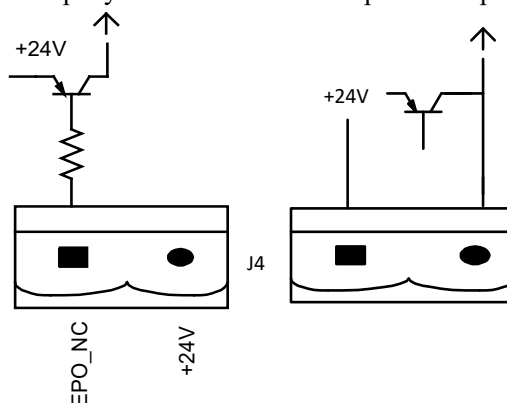
Рисунок 2-12 Схема разъема входа для дистанционного аварийного отключения питания
