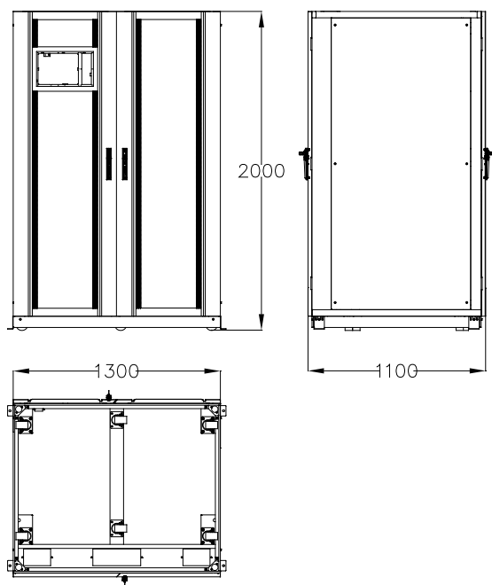
(е) Размеры для модели 400 кВА и 500 кВА (единицы измерения - мм)
