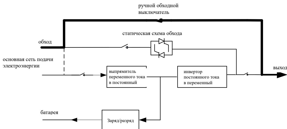
Рис. 1-б Концептуальная схема работы источника бесперебойного питания в режиме технического обслуживания
