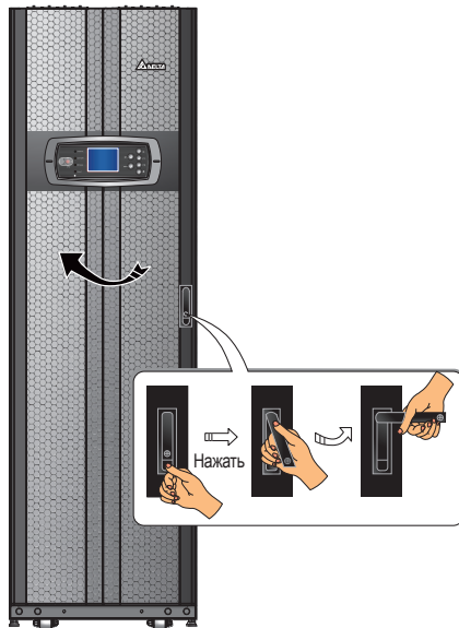
Рис. 2-4. Вид спереди
