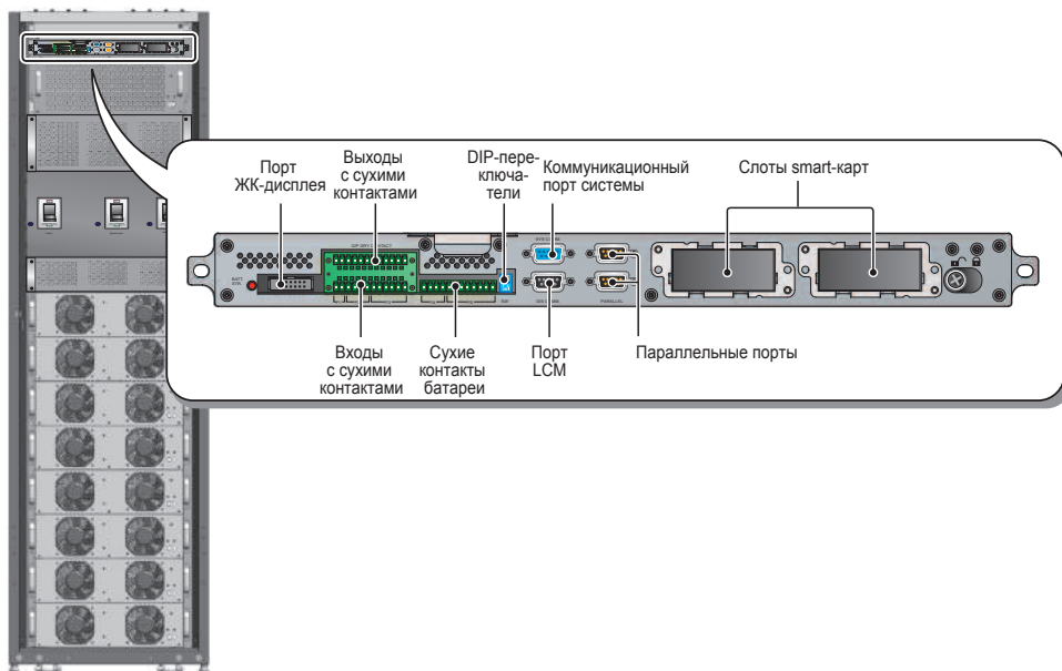
Рис. 2-12. Коммуникационные интерфейсы
