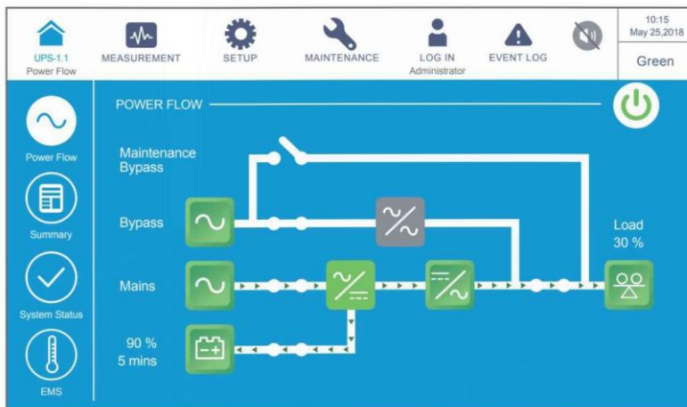
(Рисунок 6-38: Экран экологичного режима)
