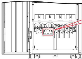
Рисунок 2-10: клеммы заземления
