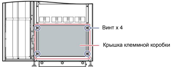
Рисунок 5-5: крышка клеммной коробки с винтами
