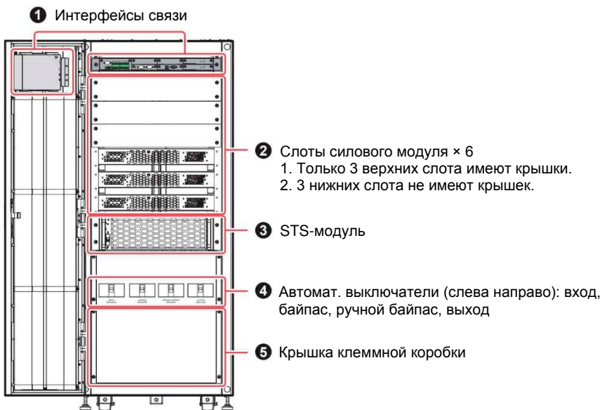
Рисунок 2-4: Шкафы ИБП внутри, передняя дверца открыта
