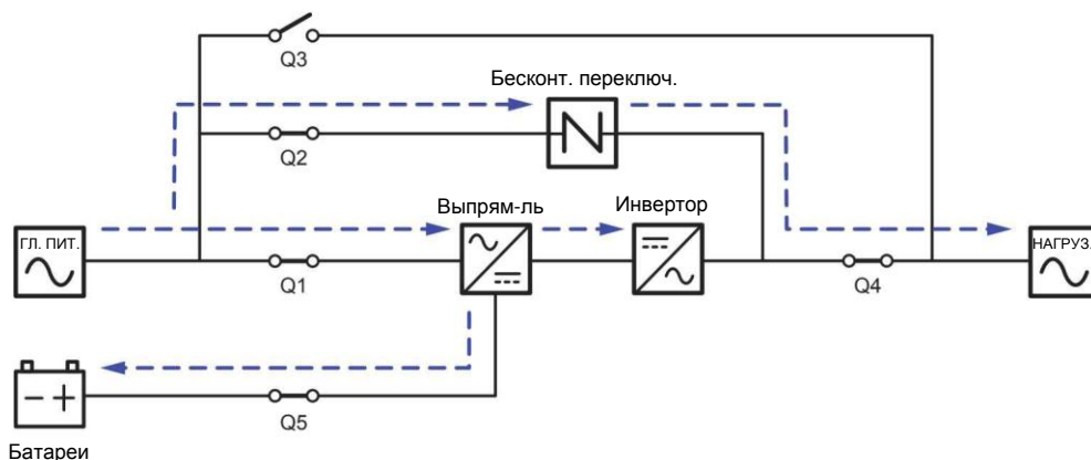
Рисунок 3-5: схема ESO-режима, подключение одного ИБП к одной линии
