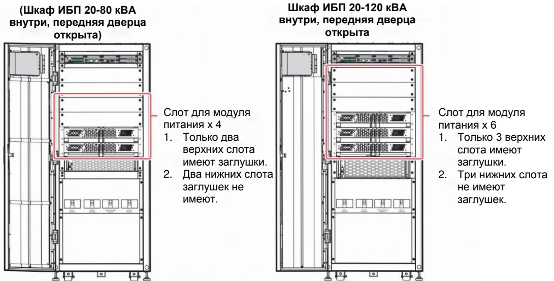
(Рисунок 5-40: Расположение заглушек слотов под силовые модули)
