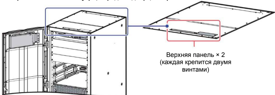
Рисунок 4-19: расположение верхних панелей
