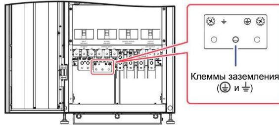
Рисунок 5-11: клеммы заземления
