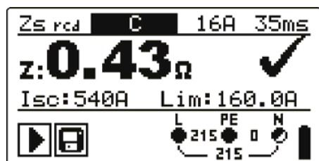
Рисунок 5.10: Примеры результатов измерения сопротивления контура
