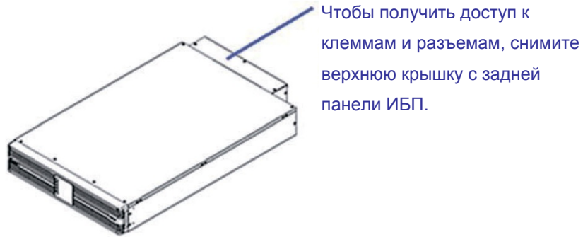
Рисунок 7-1. Расположение крышки задней панели
