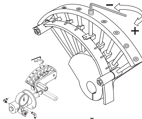
Точечная конфигурация регулировки топливо
