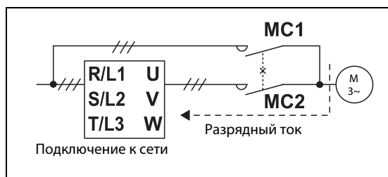
Рис. 4-1: Механическая блокировка силовых контакторов
