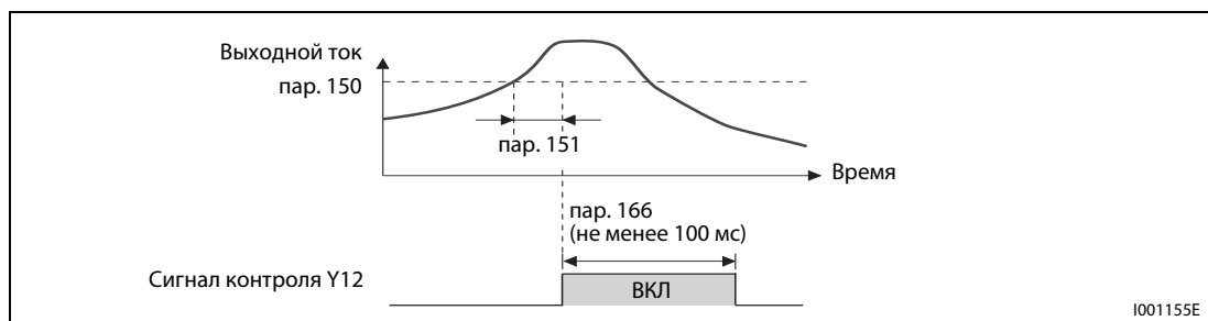
Рис. 6-55: Контроль выходного тока (пар. 166 ≠ 9999, пар. 167 = 0)
