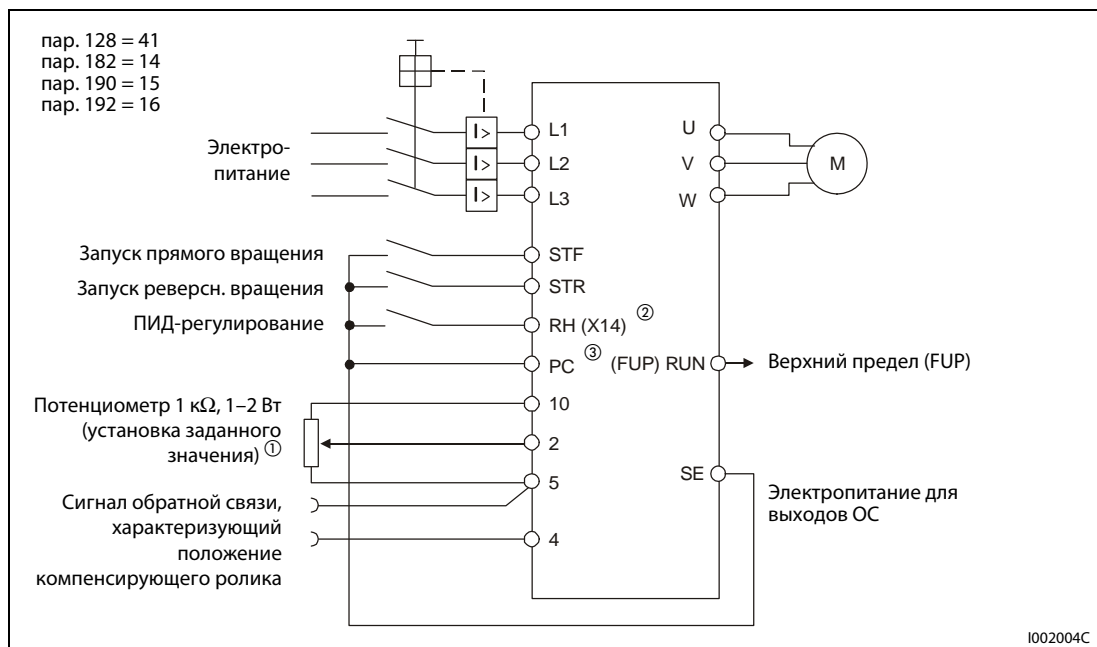
Рис. 6-132: Пример подключения при положительной логике
