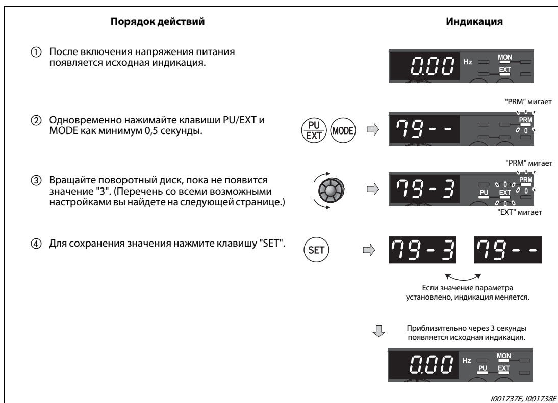
Рис. 4-8: Одновременно нажав клавиши PU/EXT и MODE, параметр 79 можно изменить сразу.
