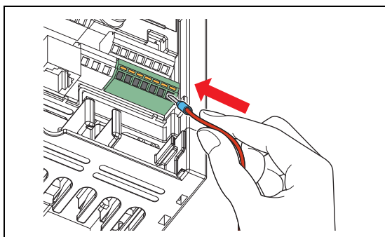
Рис. 3-10: Подсоединение провода
