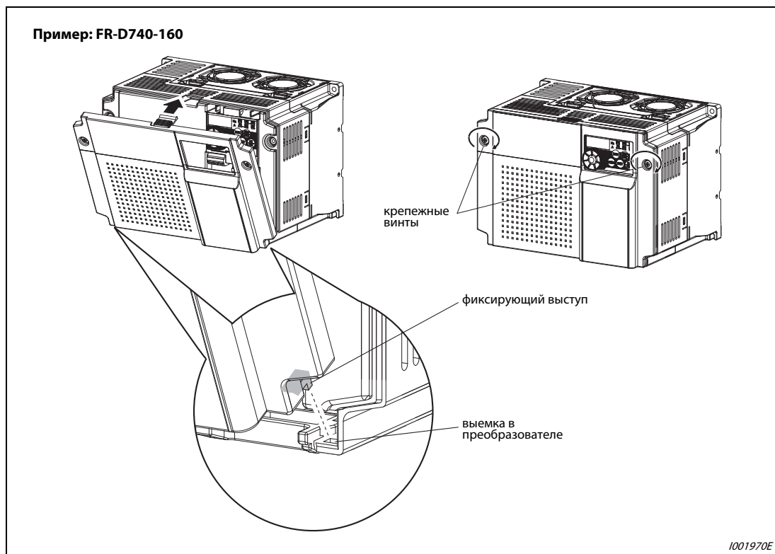
Рис. 2-4: Установка передних крышек
