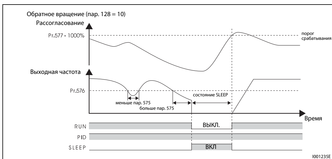
Рис. 6-126: Отключение выхода (функция SLEEP)
