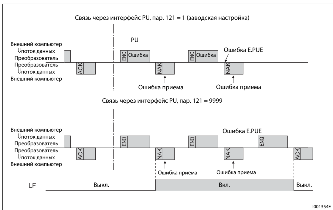
Рис. 6-103: Ошибки передачи данных
