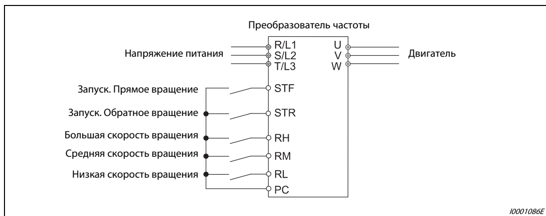
Рис. 5-22: Предустановка скорости вращения и ввод команды запуска при помощи переключателя
