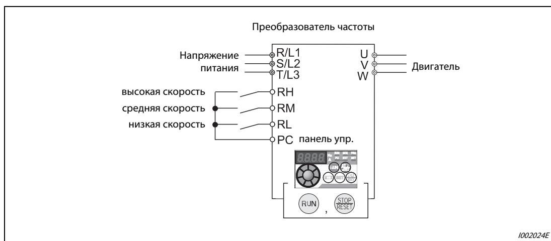
Рис. 5-13: Пример установки переключателей на клеммах RH, RM и RL
