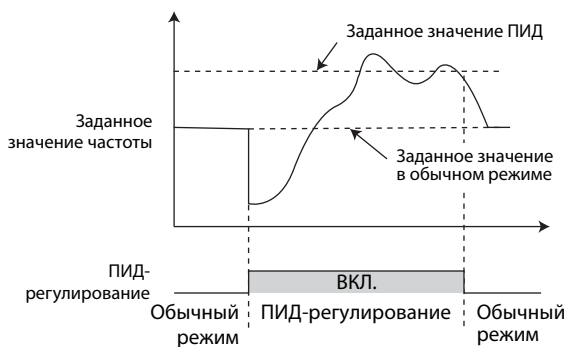
Работа при переключении с обычного режима на ПИД-регулирование
