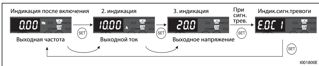
Рис. 6-59: Индикация различных рабочих параметров
