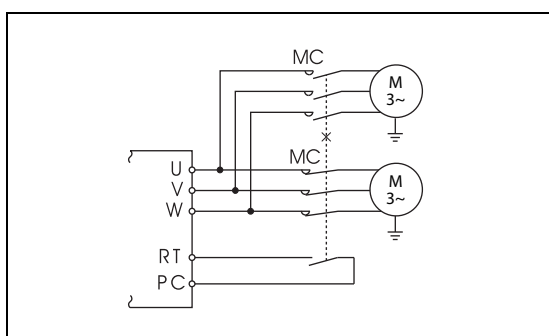
Рис. 6-34: Питание двух двигателей от одного преобразователя частоты
