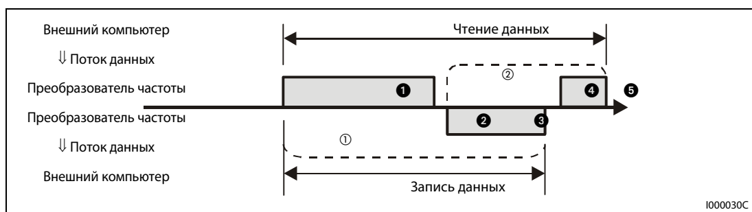
Рис. 6-108: Схематическое представление обмена данными
