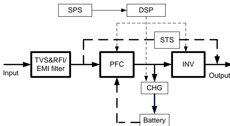
Рис. 1-3: Система ИБП
