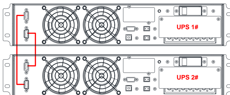
Рис. 2- 10: Параллельная система из 2 ИБП
