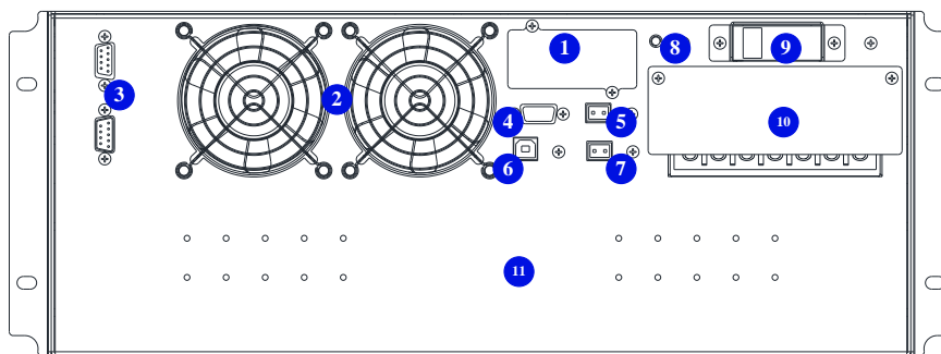
Рис 1-2: Вид задней панели 8S Power U1006RTS1, 8S Power U1006RTS1 Как показано на рисунке 1-2, задняя панель состоит из следующих компонентов и функций:
