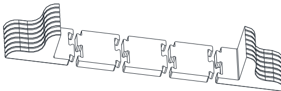
Рис.2-2 Установка опорных оснований с проставками
