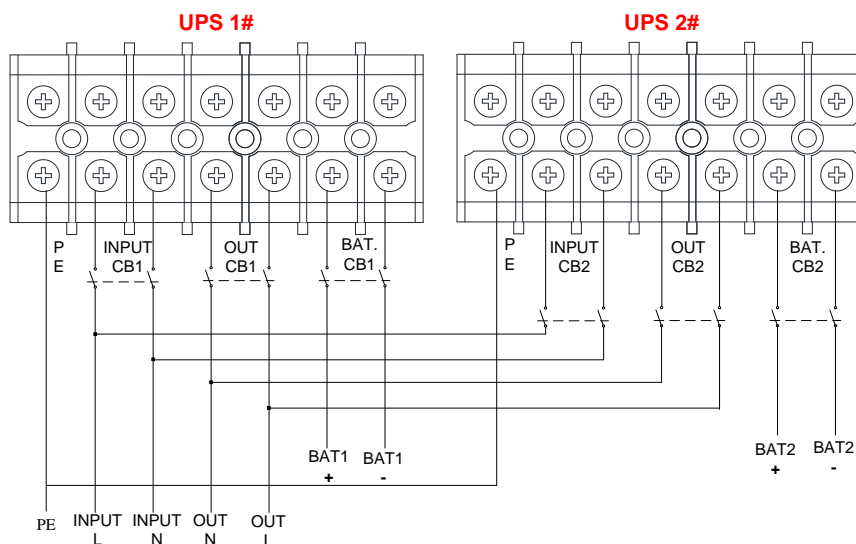
Рис. 2-9: Схема параллельного подключения
