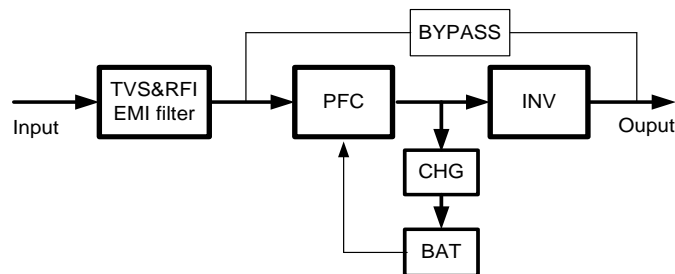
Рис. 1-4: Нормальный режим
