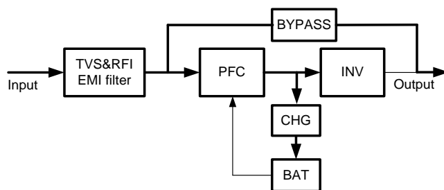
Рис. 1-7: Режим ECO
