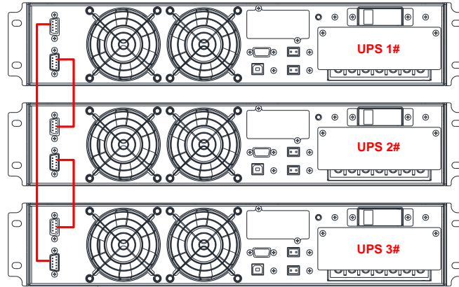
Рис 2- 11: Параллельная система из 3 ИБП
