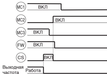
Пример переключения на питание от электросети
