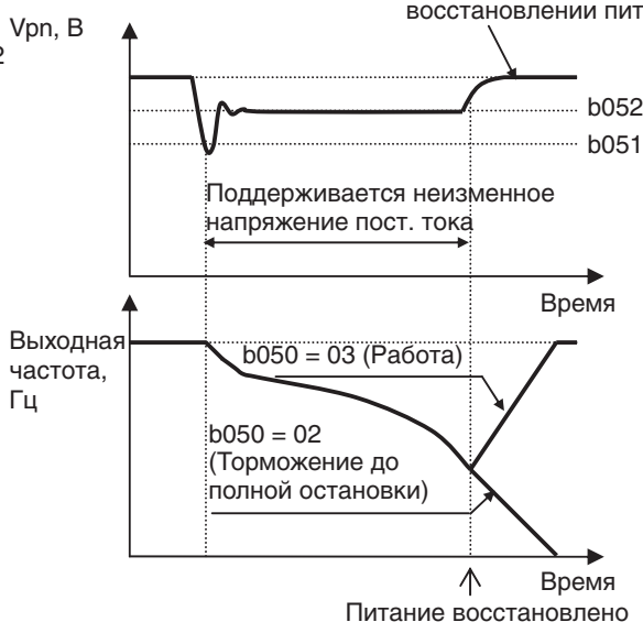
Пример 2 Напряжение силовой цепи (P-N) Напряжение шины пост. тока при восстановлении питания
