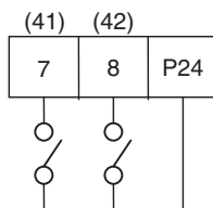
Многофункциональные входы
