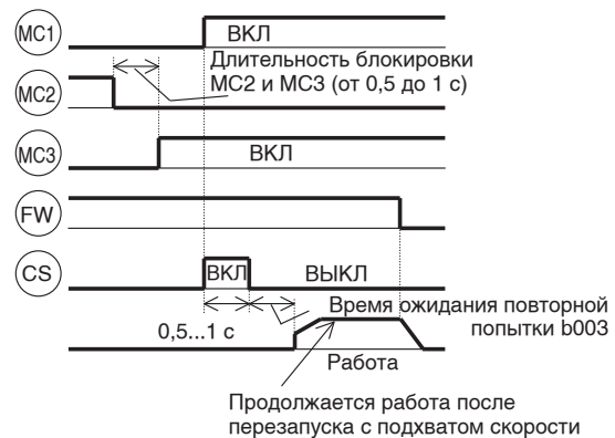
Пример переключения на питание от преобразователя частоты
