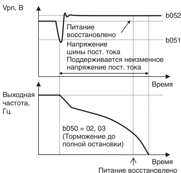
Пример 1 Напряжение силовой цепи (P-N)
