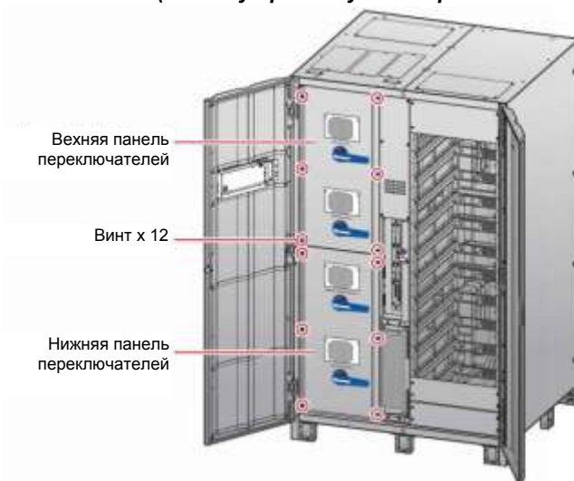
Рисунок 2-6: Расположение винтов панелей переключателей
