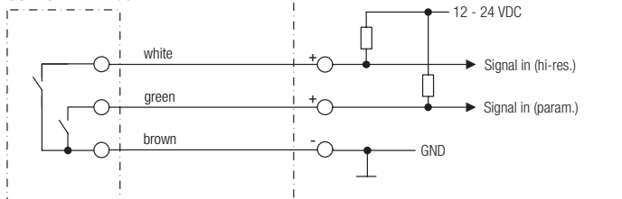
CONTOIL® VZD 4/8
