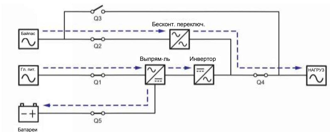
Рисунок 3-19: Схема ECO-режима, подключение одного ИБП к двум линиям питания
