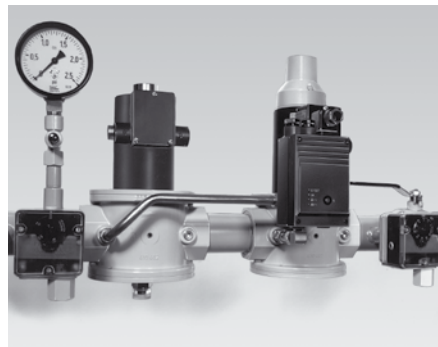
ТС 2 во входной секции между быстро и медленно открывающимися клапанами VG
