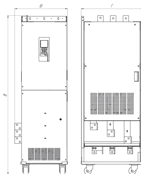
Типоразмеры 9-10 серии INPRIME
