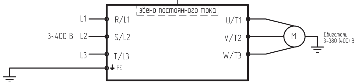
Подключение силовых клемм для моделей LCI-GY/PY-4(B)
