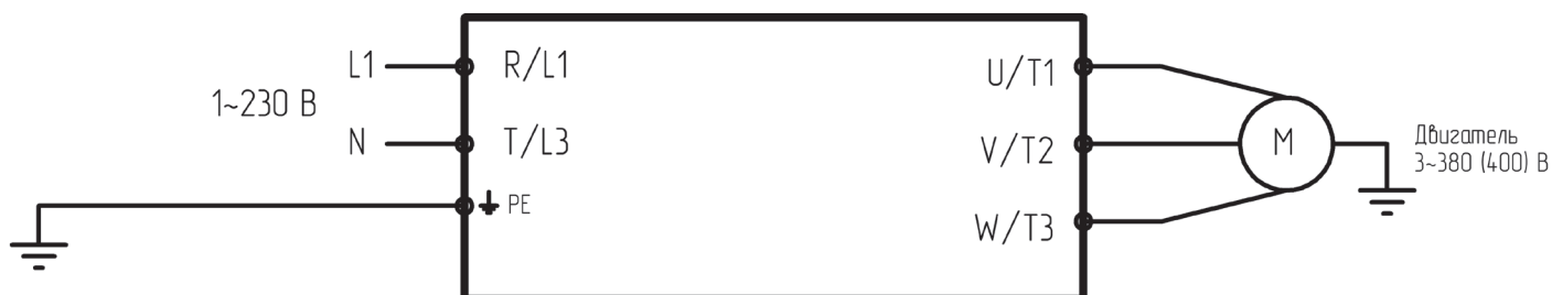
Подключение силовых клемм для моделей LCI-GY/PY-3
