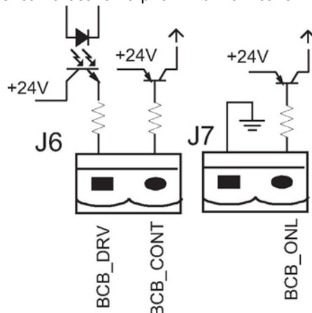
Рис. 2-10 Интерфейс ВСВ
