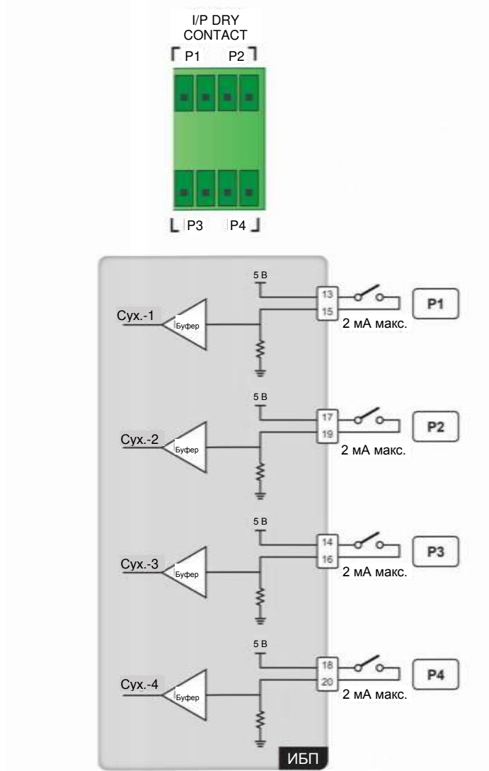
Рисунок 4-10: Схема входных сухих контактов
