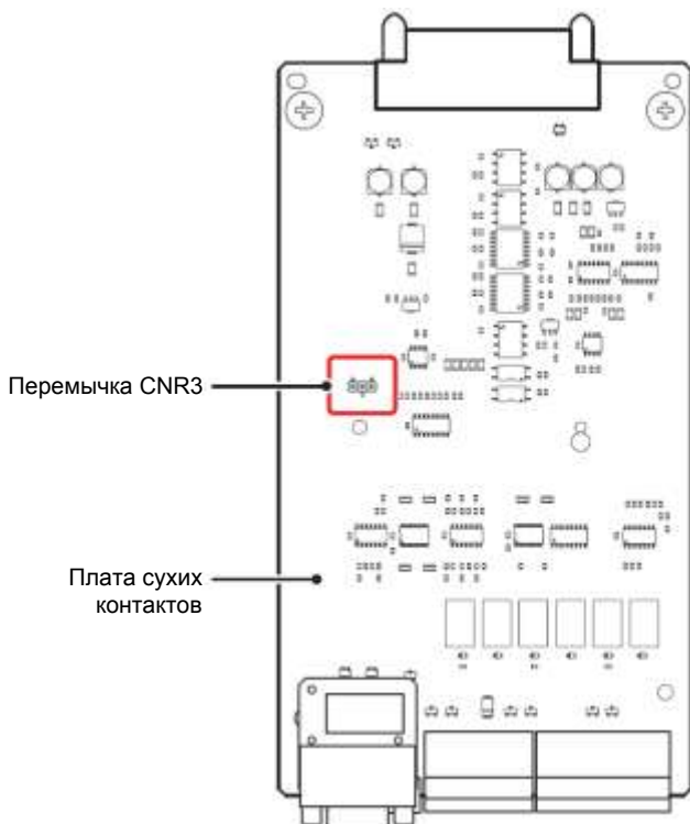
Рисунок 4-6: Расположение перемычки CNR3
