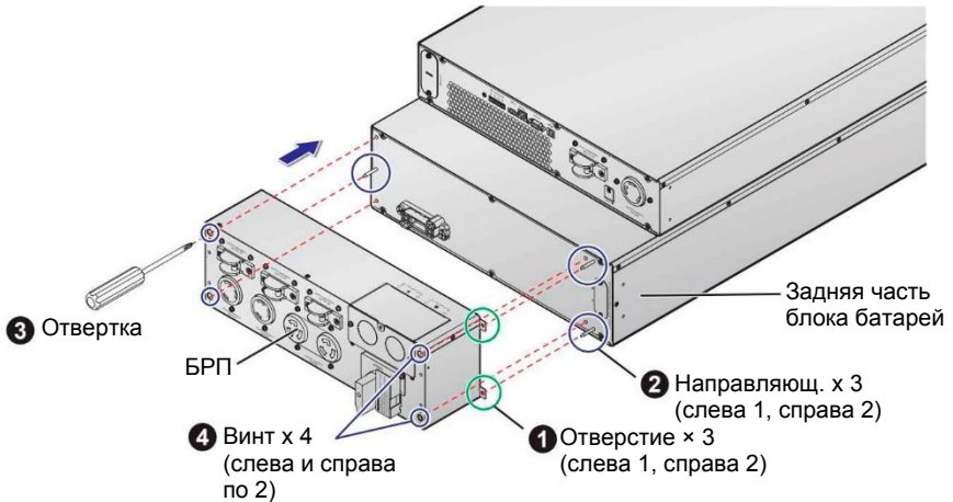
Рисунок 6-12. Монтаж БРП
