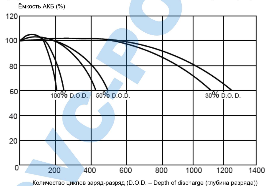
График зависимости количества циклов жизни АКБ от глубины разряда
