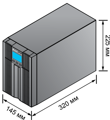
Рис. 2-1. Модель 1 кВА, внешний вид и размеры
