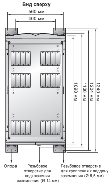
Рис. 2-3. Расположение крепежных отверстий
