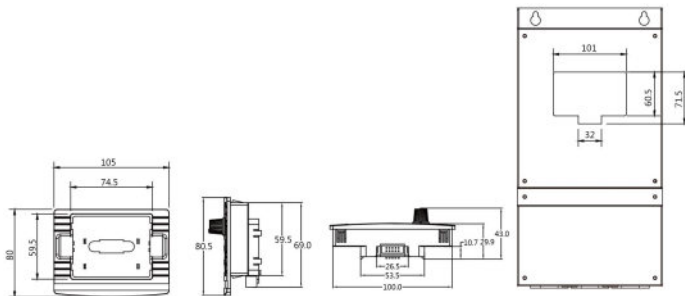
Основание клавиатуры
