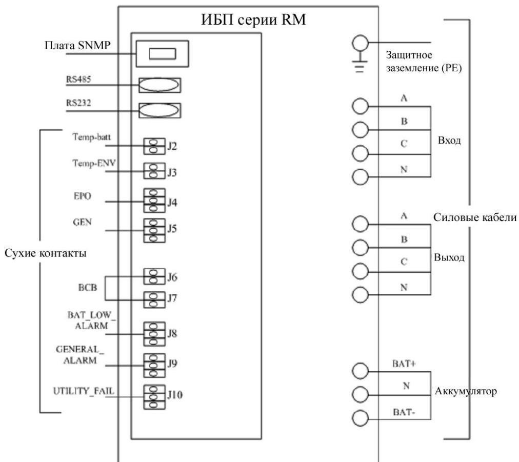
Рис. 1-21. Схема установки
