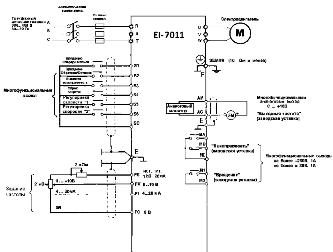
Рис. 9. Схема подсоединения.
