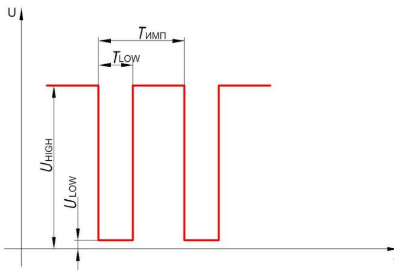
Рис.3. Вид выходного сигнала EUROSENS X PN(RS) Z V(Характеристики приведены в таблицах 10,11)
