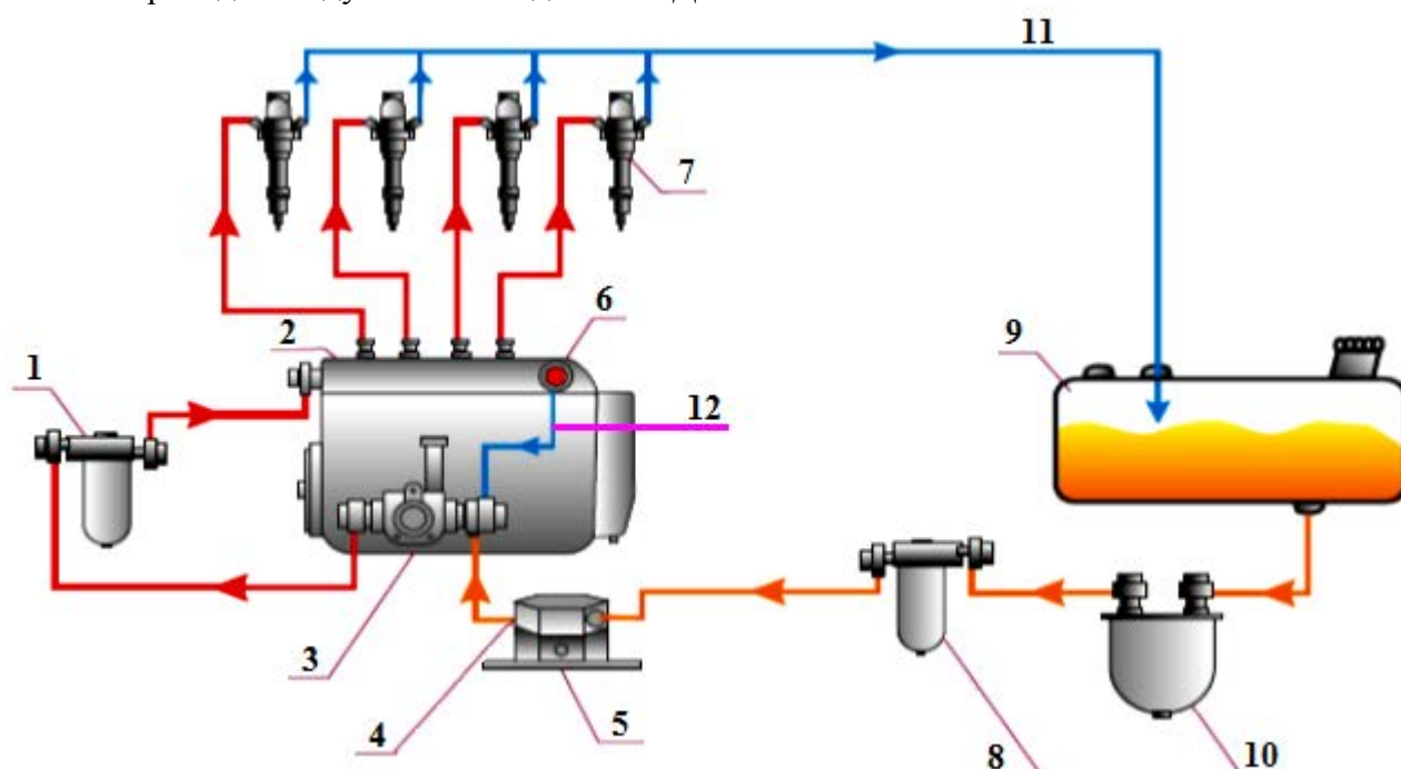
Рис.6. Схема установки датчика Direct "На разрежение" с подкачивающим насосом низкого давления
