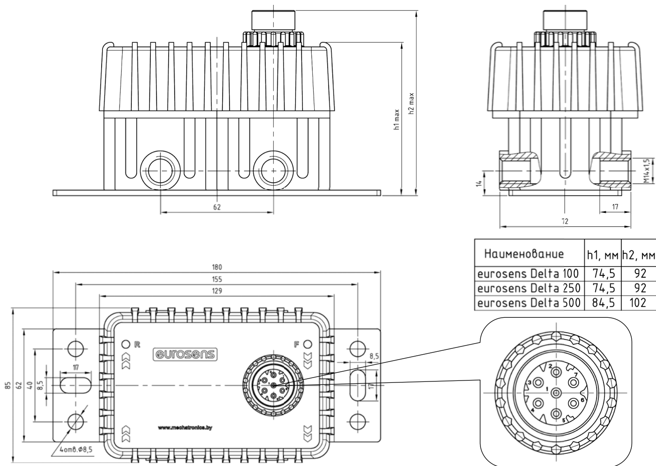
Рис.17. Габаритные и установочные размеры EUROSENS Delta PN (RS) , где F – Forward/Подача, R – Return/Возврат
