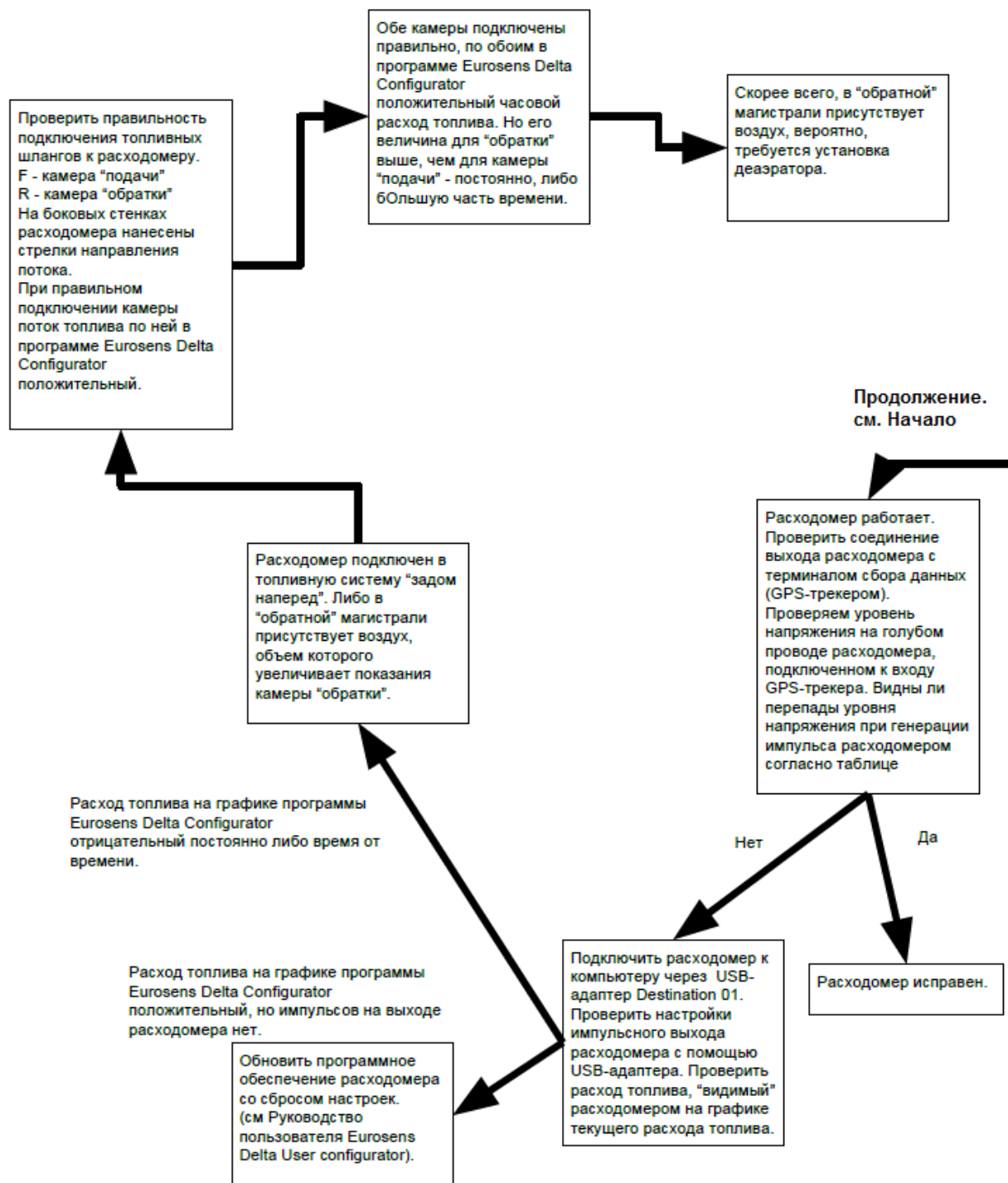
Рис.15. Экспресс-диагностика датчиков расхода EUROSENS Delta (Продолжение)
