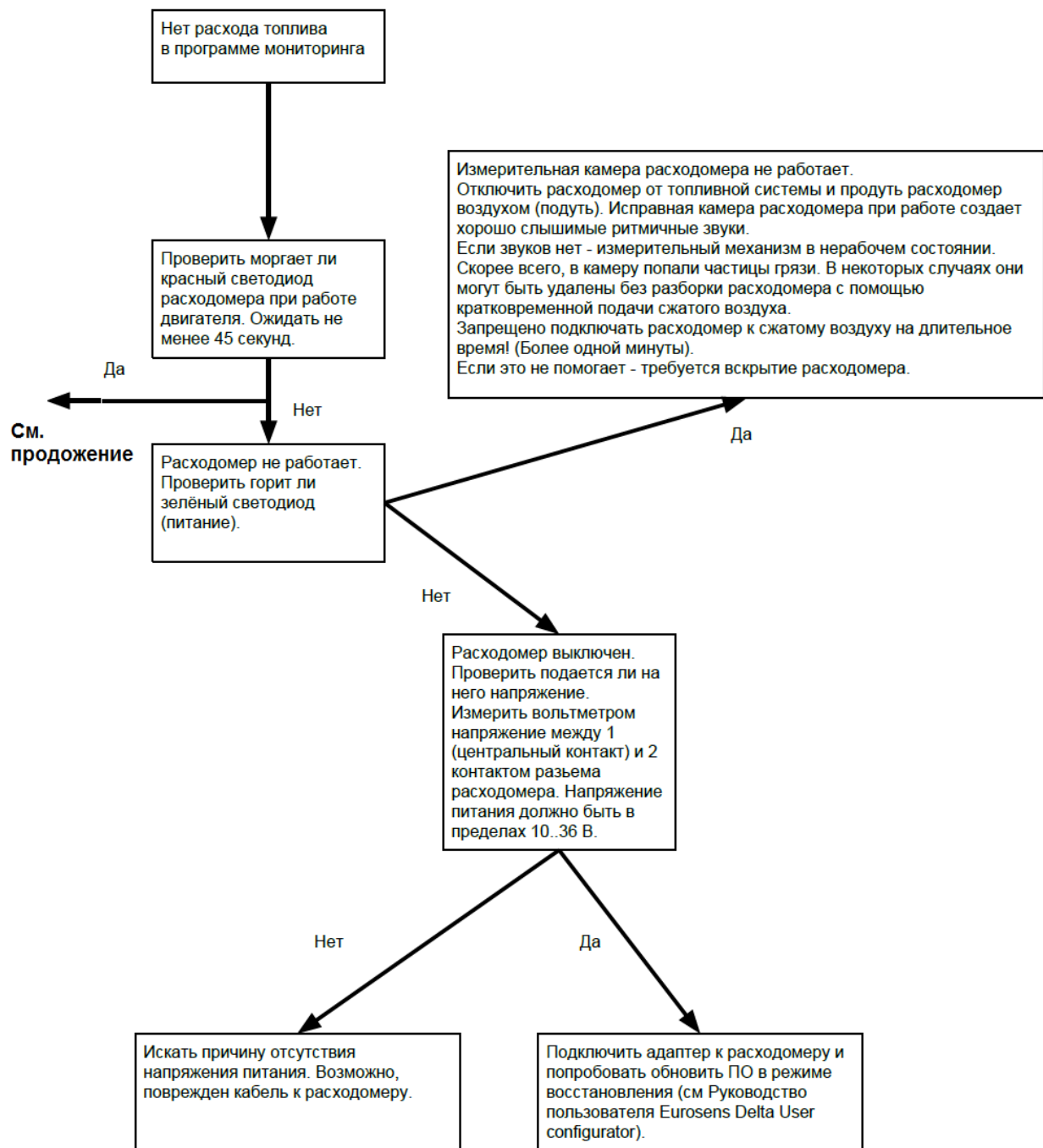
Рис.12. Экспресс-диагностика датчиков расхода EUROSENS Direct (Начало)
