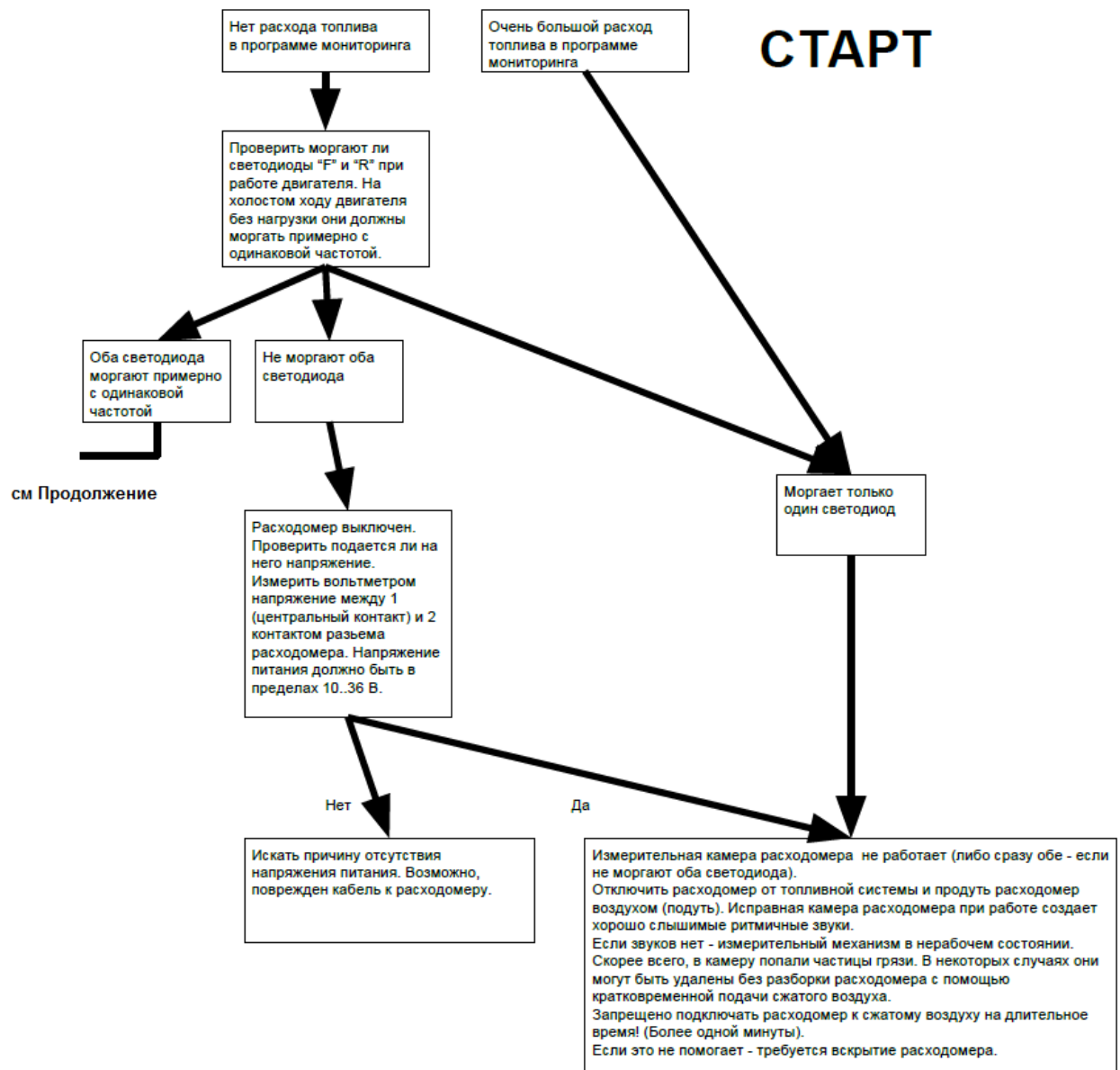
Рис.14. Экспресс-диагностика датчиков расхода EUROSENS Delta (Начало)
