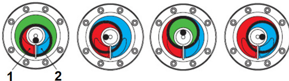
Рис. 1. Схема работы измерительной камеры EUROSENS ,
