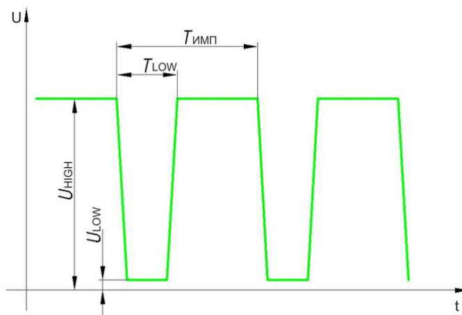
Рис. 2. Вид выходного сигнала EUROSENS X P(PH) Z V(Характеристики приведены в таблицах 10,11),
