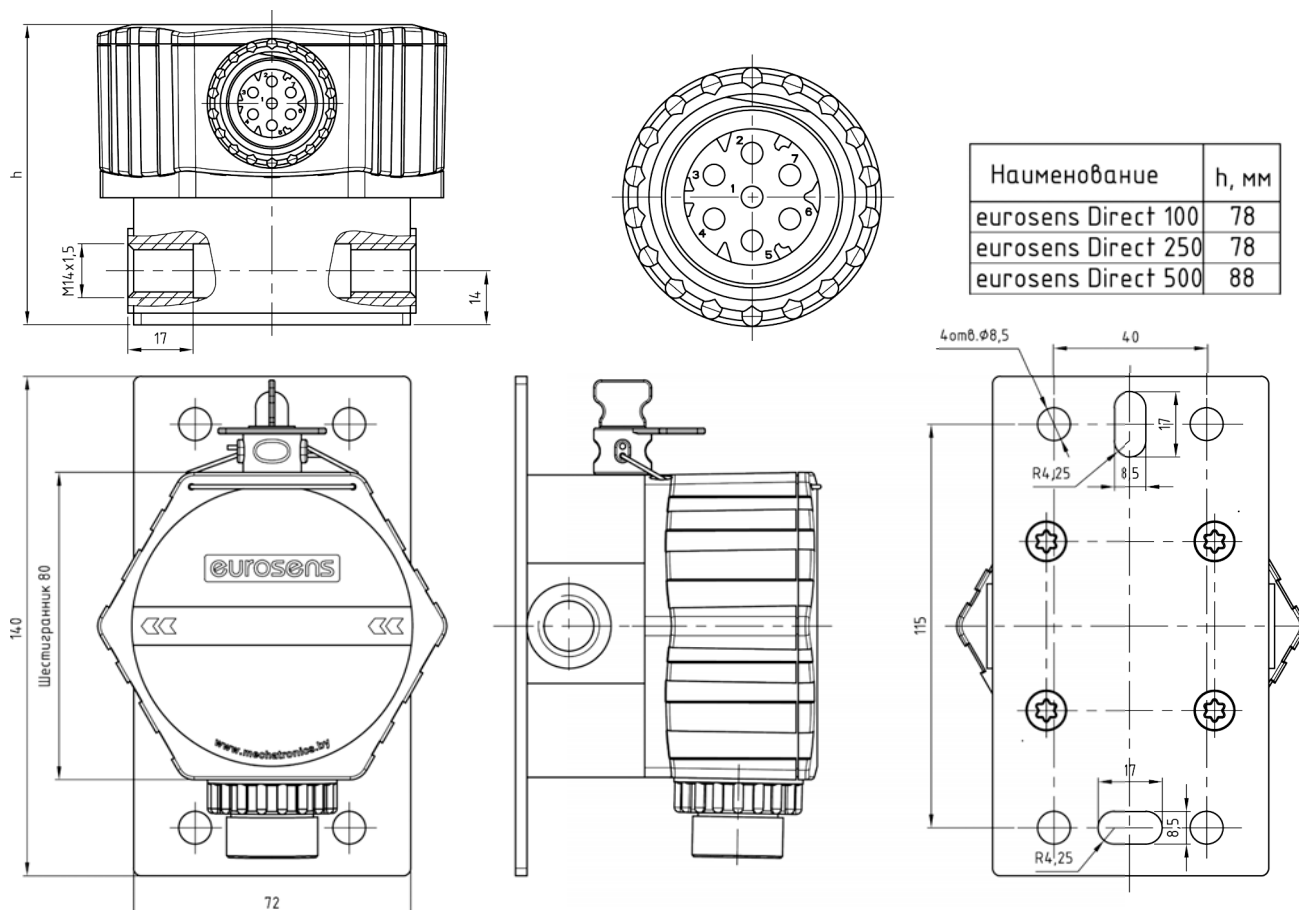
Рис.16. Габаритные и установочные размеры EUROSENS Direct P (PH, PN, RS)
