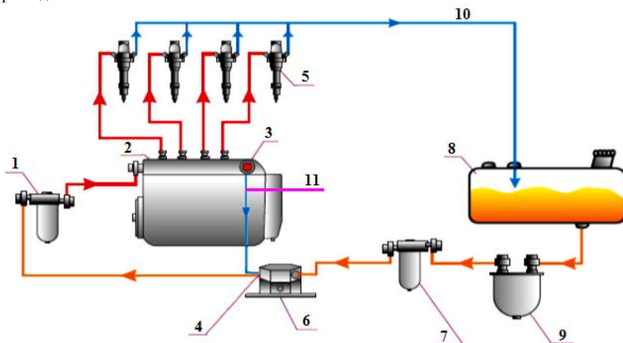
Рис.7. Схема установки датчика Direct "На разрежение" без подкачивающего насоса низкого давления
