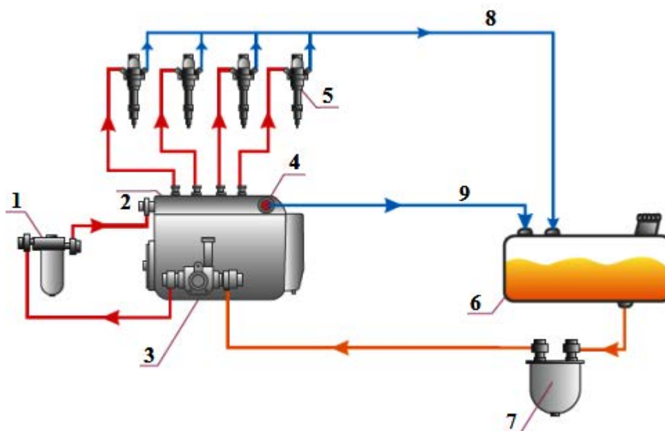
Рис.4. Типовая схема топливной системы
